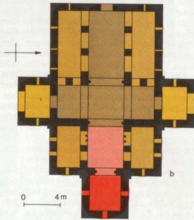
El Campillo: San Pedro de la Nave, 7. Jh. a Ansicht von NO b Grundriß
