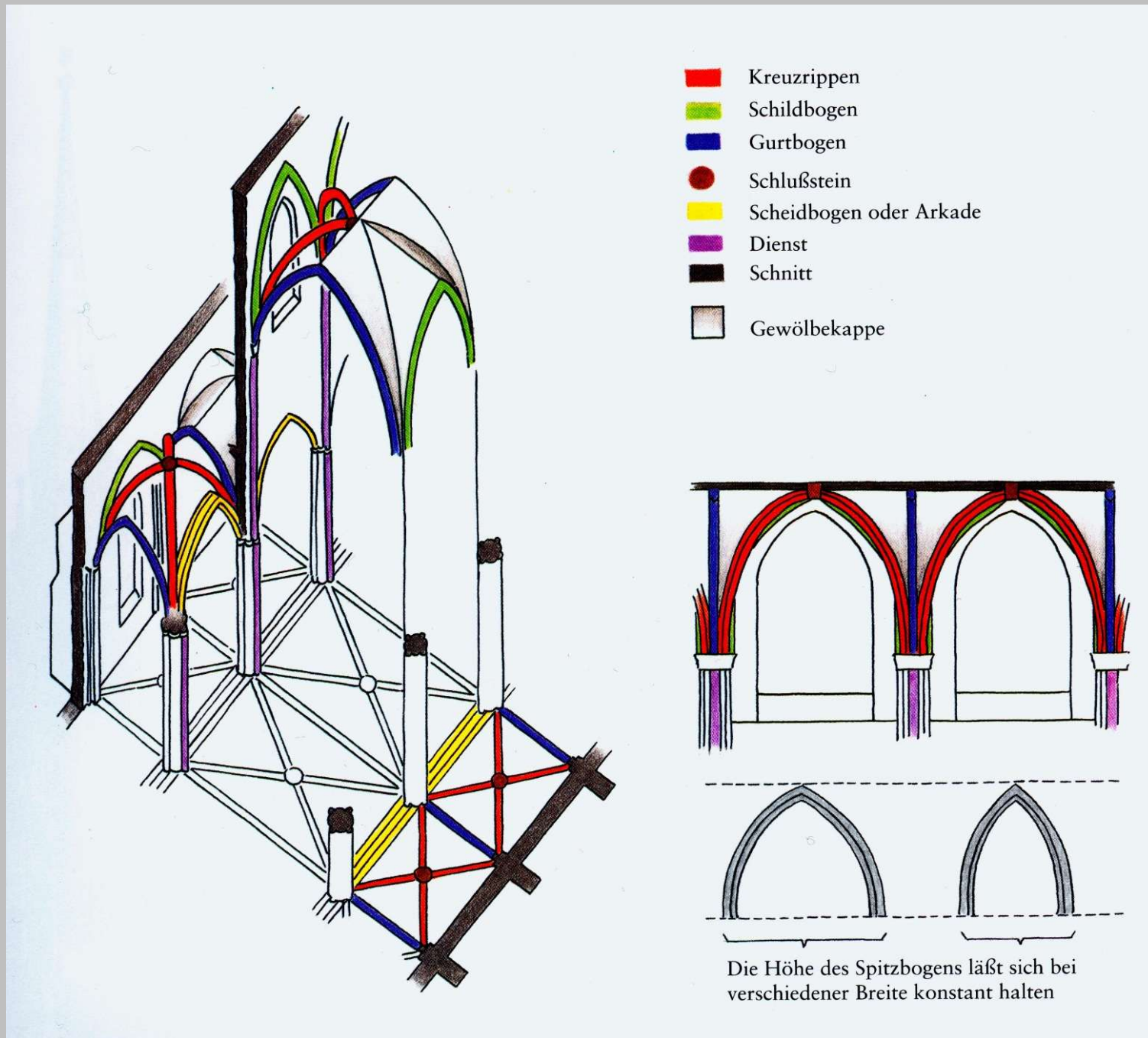
Spitzbogen und Kreuzgewölbe
