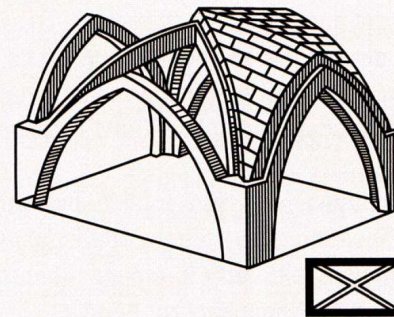
Kreuzrippen- gewölbe
