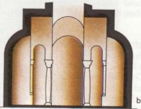
Mailand: Kapelle bei San Satiro a Grundriß b Schnitt 0 4m
